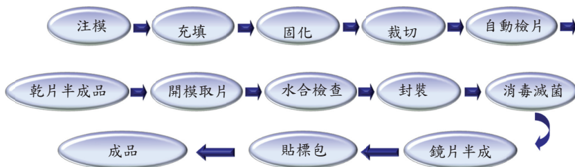
拋棄式鏡片生產流程
