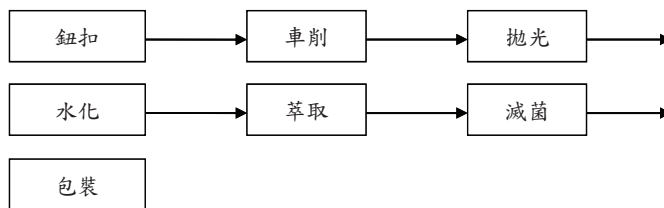
傳統車削軟式鏡片生產流程
